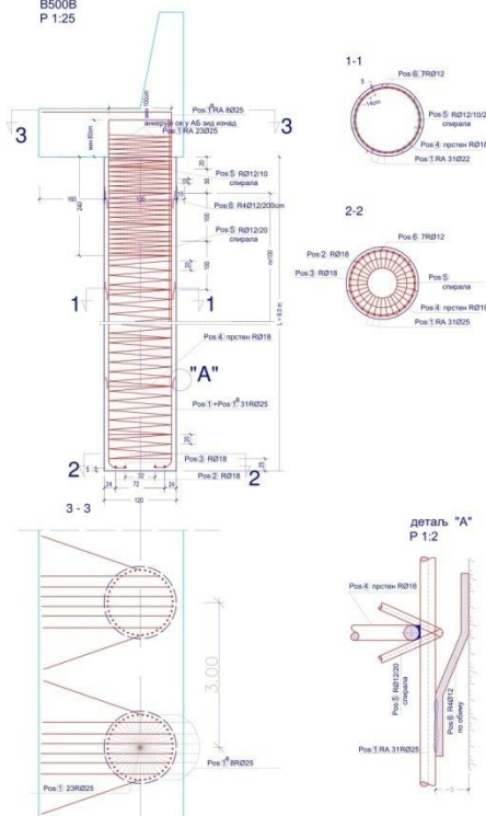
ПЛАН АРМАТУРЕ ШИПОВА ИСПОД ЗИДА Ø1200мм, L=9.00m C30/37 B500B P 1:25
